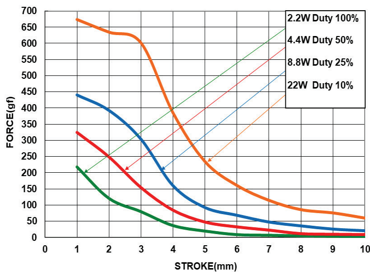
Kraft-Wege-Diagramm / Stroke-Force-Diagram
